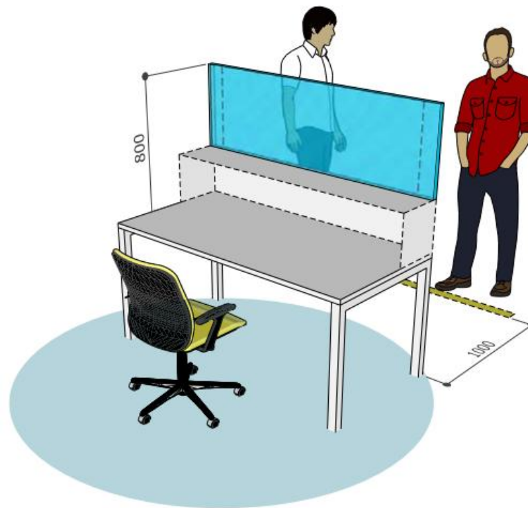
Figura 14 - Postazione front office o banco reception - visitatori in piedi
