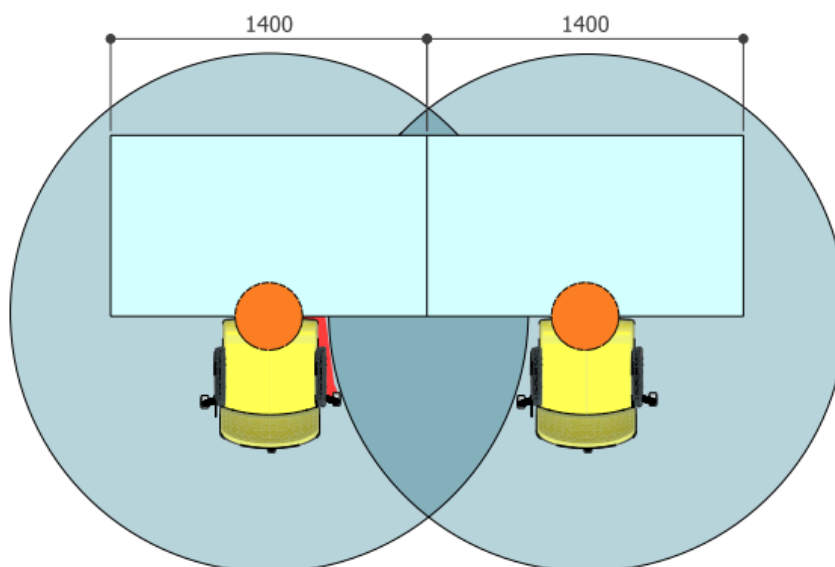
Figura 8 - Scrivanie da 1400 mm affiancate sul lato corto
