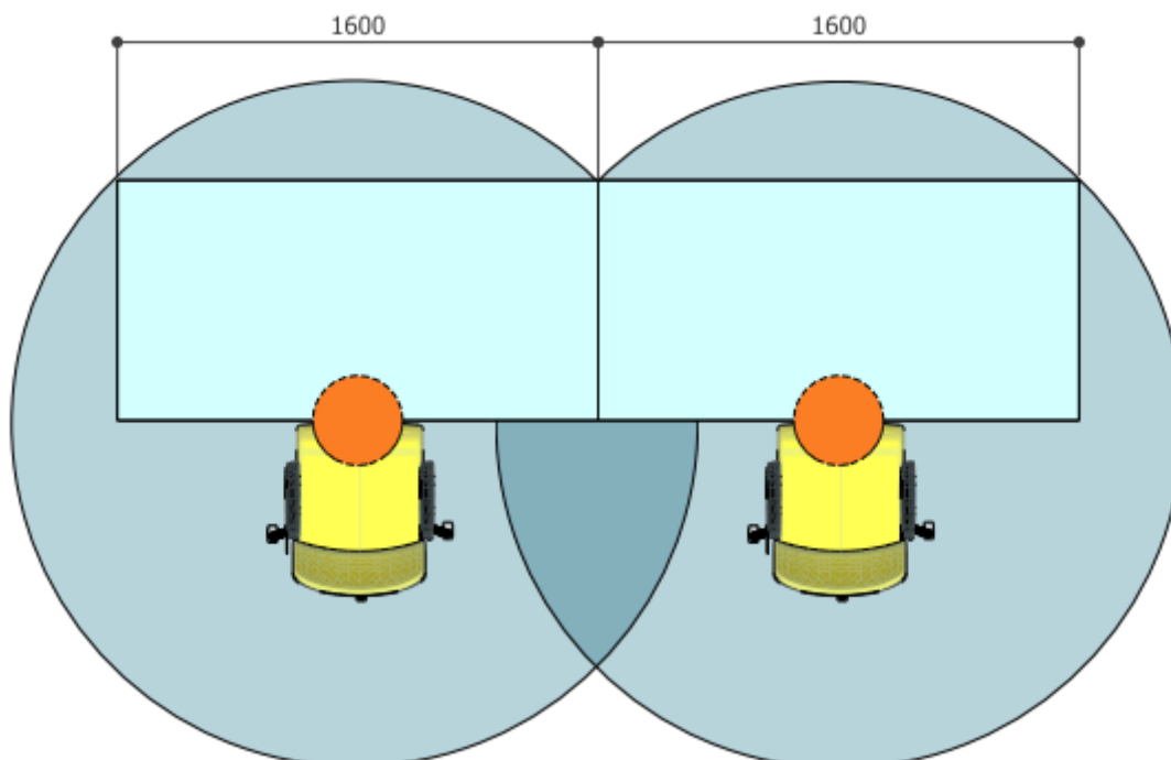
Figura 3 - Scrivanie da 1600 mm affiancate sul lato corto
